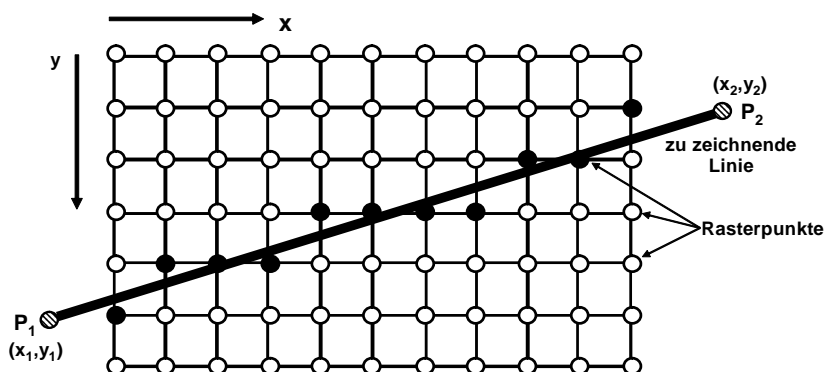
Abb. 11.1: Zeichnen einer gerasterten Linie
