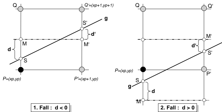
Abb. 11.2: Mittelpunkts-Algorithmus von Bresenham
